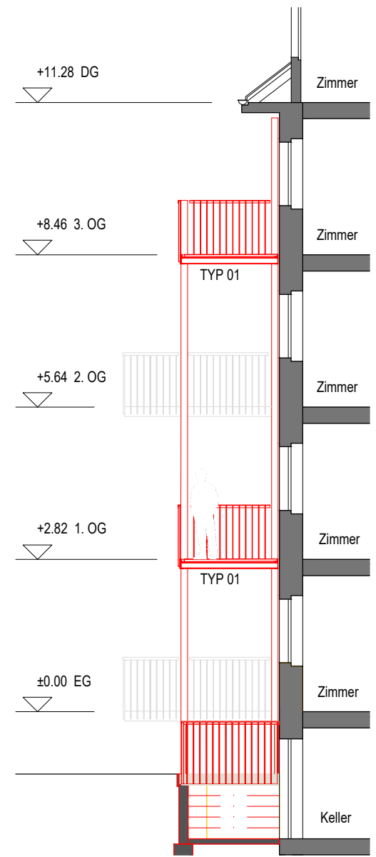
SCHNITT A-A
