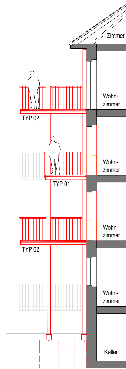
SCHNITT B-B
